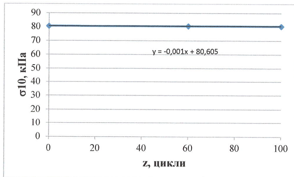
Рисунок 6 – Залежність міцності на стиск при 10% деформації від циклічних впливів зразків теплоізоляційного матеріалу марки «ТЕХНОРУФ ПРОФ»
